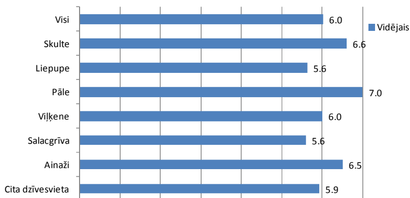
Lūdzu, novērtējiet, cik svarīgi Jūsu teritorijas attīstībai bija realizēt projektus../ 5.1.1. Teritorijas dzīves vides kvalitātes uzlabošana. Novērtējums skalā līdz 7, kur 1 ir mazsvarīgi,
