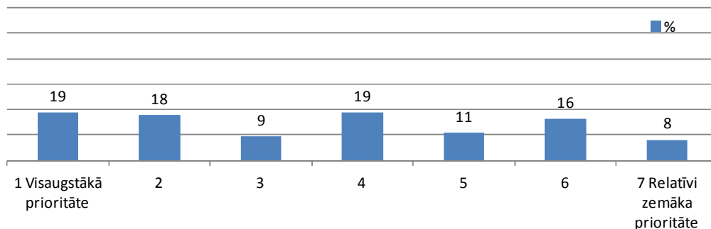
3.1. Lauksaimniecības produktu ražošana un pirmapstrāde. Sarindojiet prioritāšu secībā (1 – visaugstākā prioritāte, 7 – relatīvi zemāka prioritāte)
